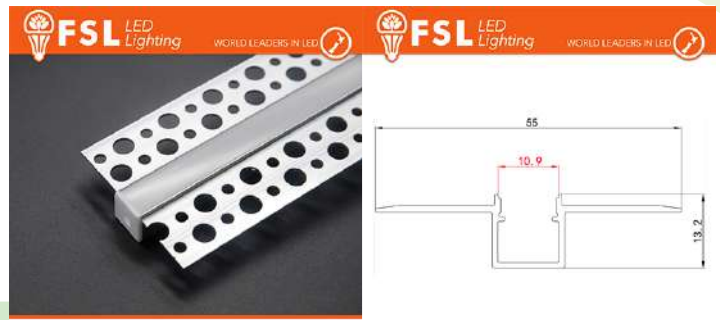
Profilo Alluminio
